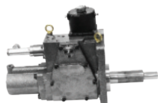
260 REG ASS'Y
